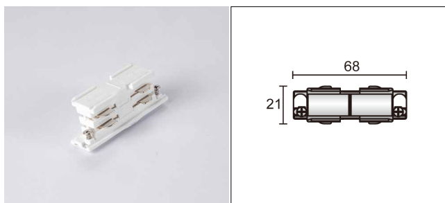
Mini joiner
